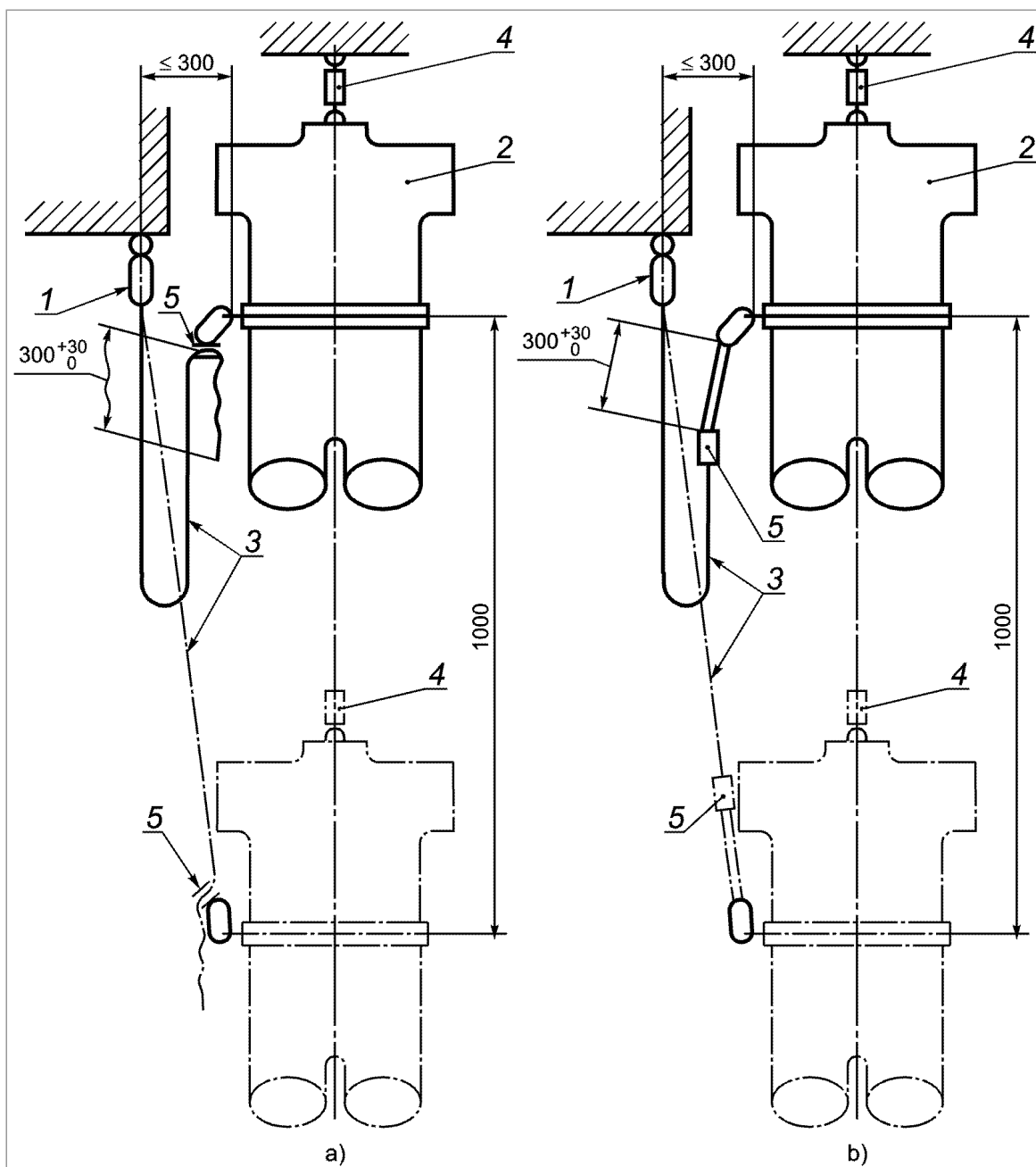
Рисунок 10 - Испытание на динамическую прочность поясного ремня со встроенным стропом фиксированной длины
